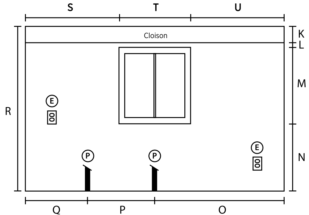
Plan d'élévation du mur (Vue de face)
